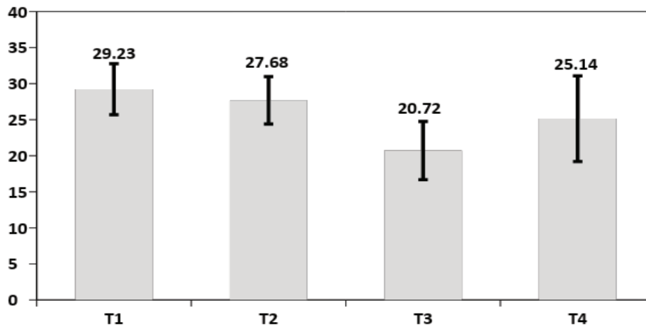
Figura 6. Resistência a compressão aos 14 dias de cura seca.
